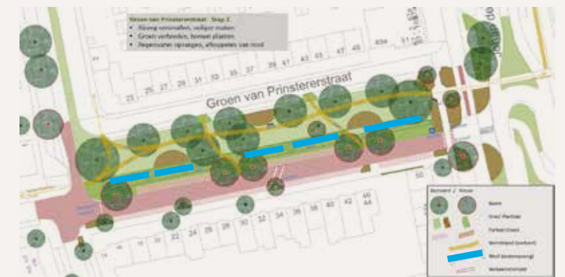
Uitvoering fase 2: 950 m2 onttegen – versmallen rijweg, open verharding parkeerplaatsen, verwijderen trottoir – extra bomen, wadi, afkoppelen, padden halfverharding, bloemenvelden
